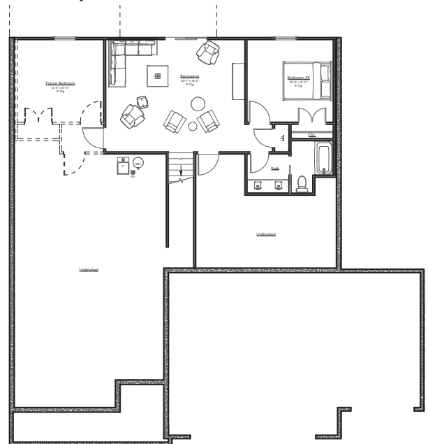
Optional Lower Level
